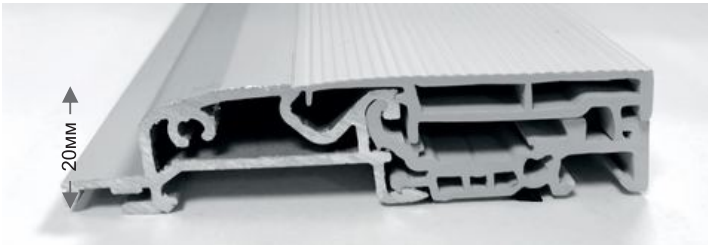
Drempelloze originele VEKA Softline-dorpel van 20 mm hoog, met een thermische onderbreking van kunststof die indien nodig eenvoudig te vervangen is.
