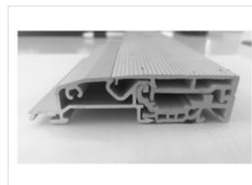
Thermisch stabiele originele VEKA-dorpel 20 mm met kunststof opzet en waterkering
