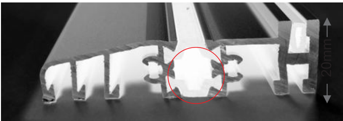
Aluminium dorpel met thermische onderbreking beperkt de kans op bevrozing in de winter.
