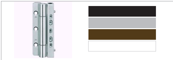
Simonswerk-scharnieren met inbraakwerende pen zijn in drie richtingen verstelbaar en lopen op glijlagers — betrouwbaar en onderhoudsvrij.
